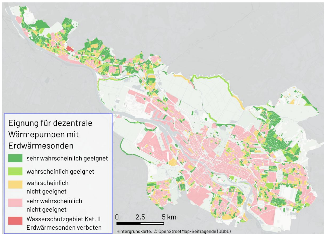
Abbildung 108: Eignungsstufen für die Wärmeversorgung mit dezentralen Sole-Wasser-Wärmepumpen mit Erdwärmesonden nach Baublöcken in Bremen im Zielszenario gemäß § 19 WPG, unter Berücksichtigung des durch Sanierung reduzierten Wärmebedarfs
