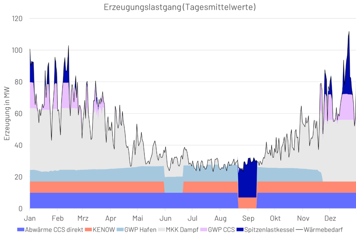
Abbildung 76: Erzeugersimulation Netzgebiet West für das Zielszenario
