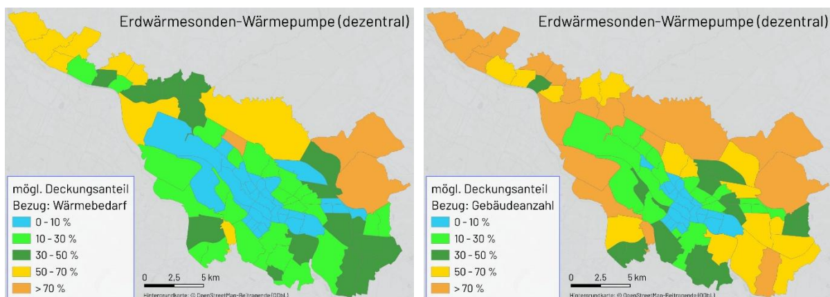
Abbildung 60: Mögliche Deckung mit dezentralen S/W-WP mit Erdwärmesonden in den Ortsteilen von Bremen nach energetischer Sanierung mit Reduktion des heutigen Bedarfs auf 50 %: (links) bezogen auf den Wärmebedarf, (rechts) bezogen auf die Gebäudeanzahl.
