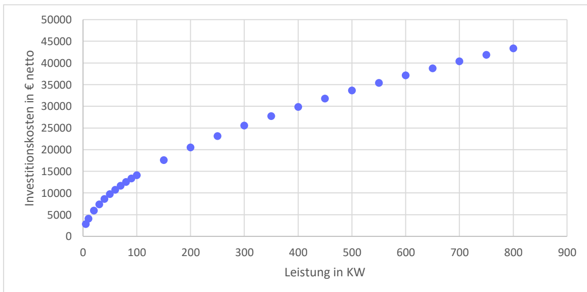
Abbildung 68: Kostenannahme für Hausanschlussstationen
