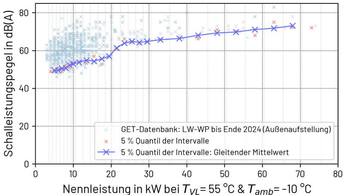
Abbildung 49: Zusammenhang zwischen der Schalleistung von L/W-WP und der Heizleistung, basierend auf Datenblattwerten aus der GET-Produktdatenbank (Amt der Salzburger Landesregierung - Lebensgrundlagen und Energie, 2023). Die angesetzte Funktion orientiert sich an den emissionsärmsten Wärmepumpen der jeweiligen Leistungsklasse.
