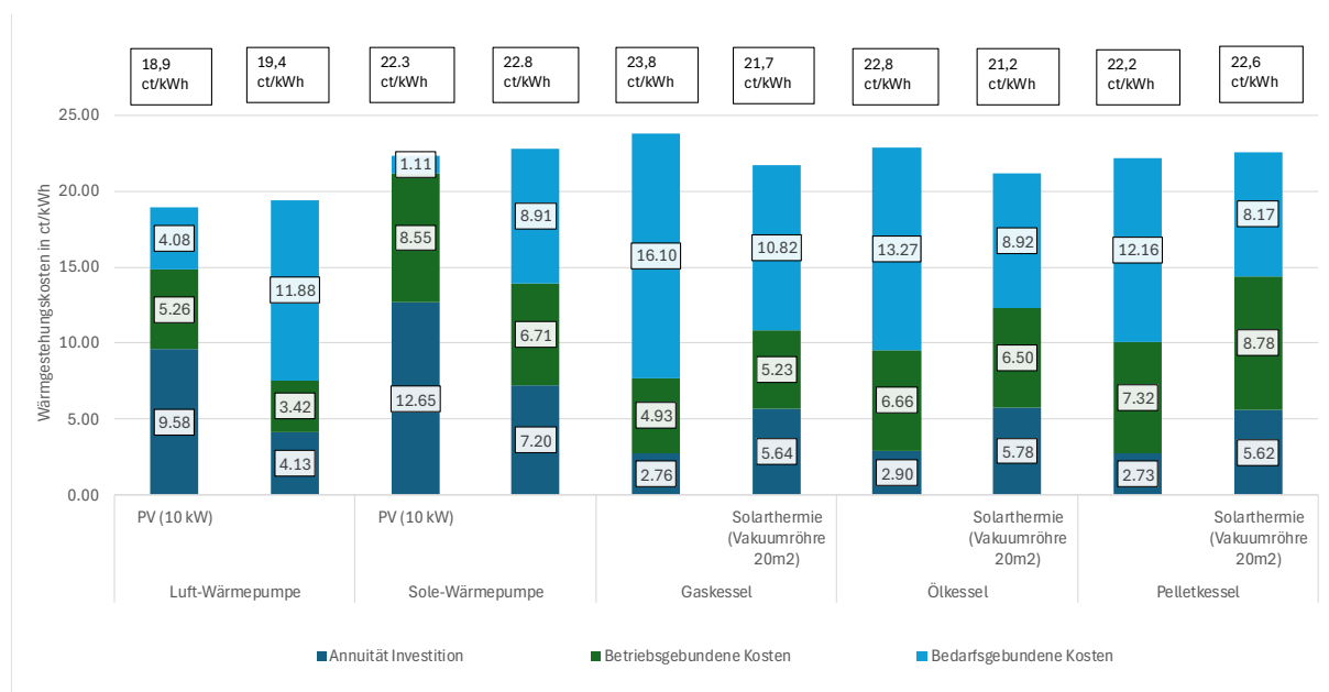
Abbildung 110: Netto-Wärmegestehungskosten für Heizleistungen von 12 kW für dezentrale Wärmeerzeugungsmethoden
